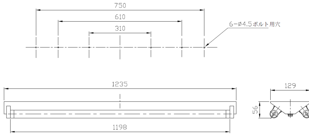
LEDランプ外形寸法
